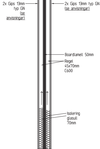
SNITT A-A
