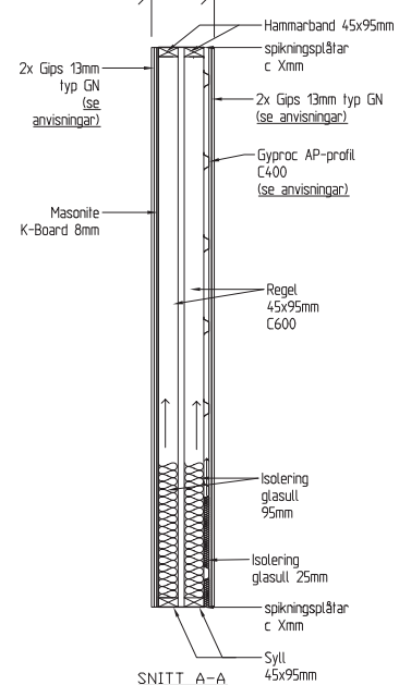
SNITT A-A
