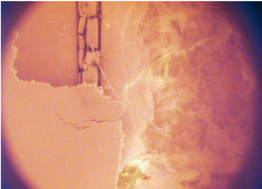
Från fönster i brandprovningssugn. Brinnande träregel i mitten, delvis skyddad med gipsskiva. Icke-högvärmebeständig mineralull till höger och högvärmebeständig mineralull till vänster.
